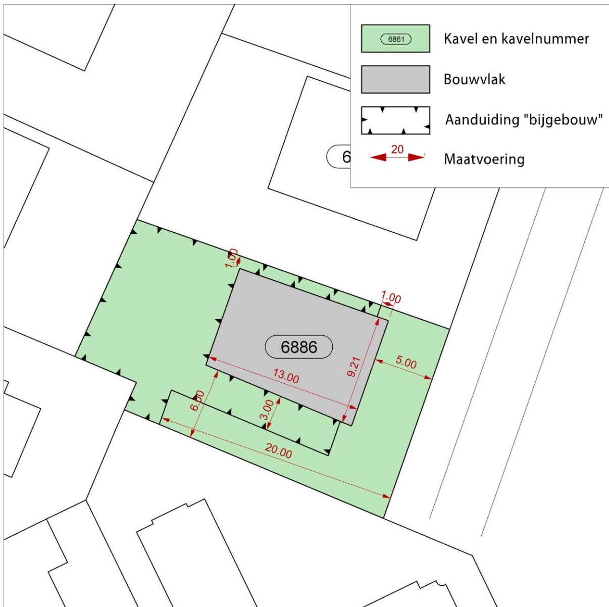
Afbeelding 4: bebouwingsgrenzen geprojecteerd op kavel 6886.
