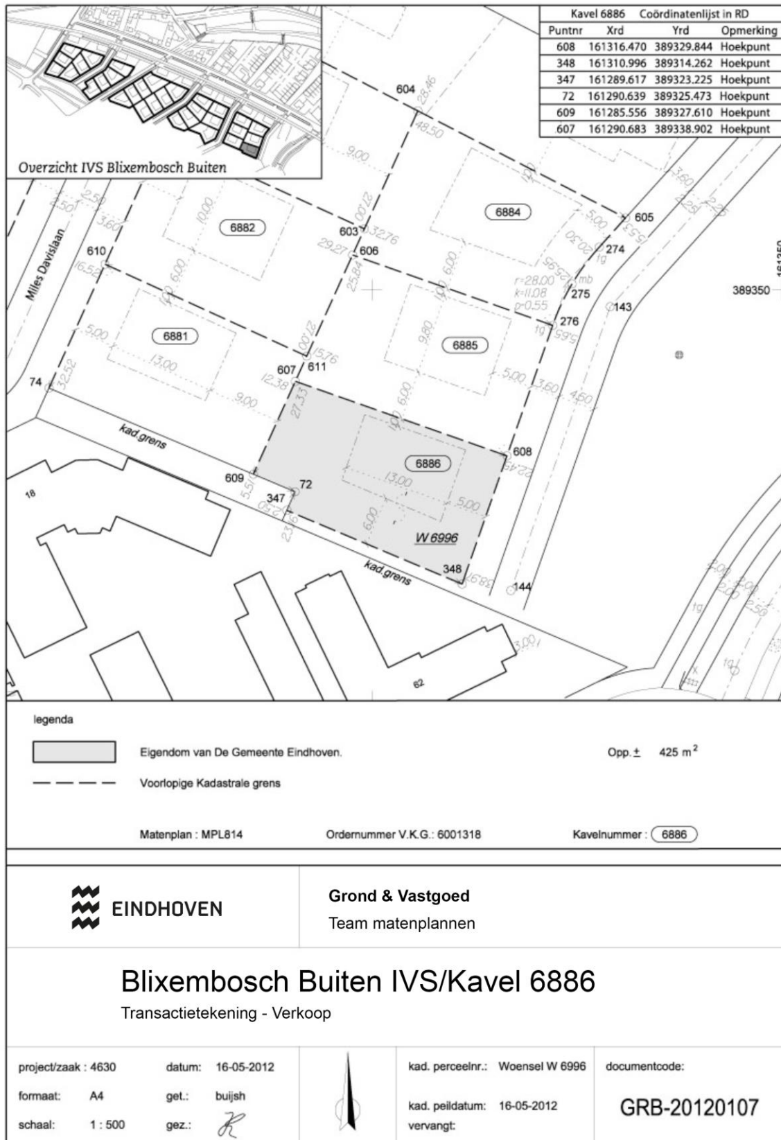
Afbeelding 3: Kadastrale verkooptekening van kavel 6886.
