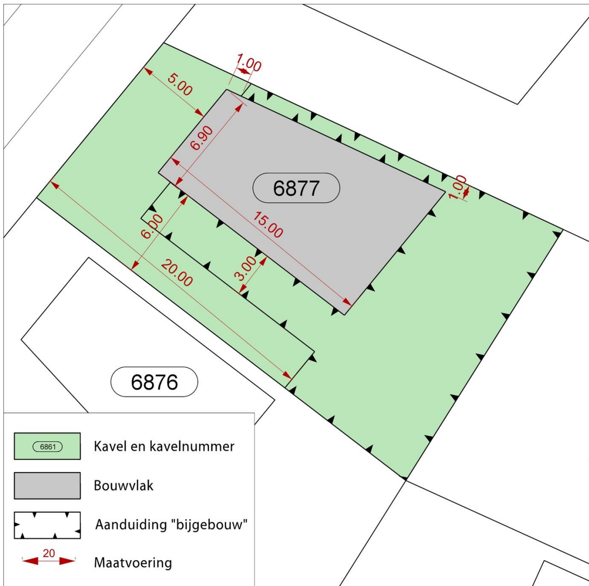
Afbeelding 4: bebouwinggrenzen geprojecteerd op kavel 6877.
