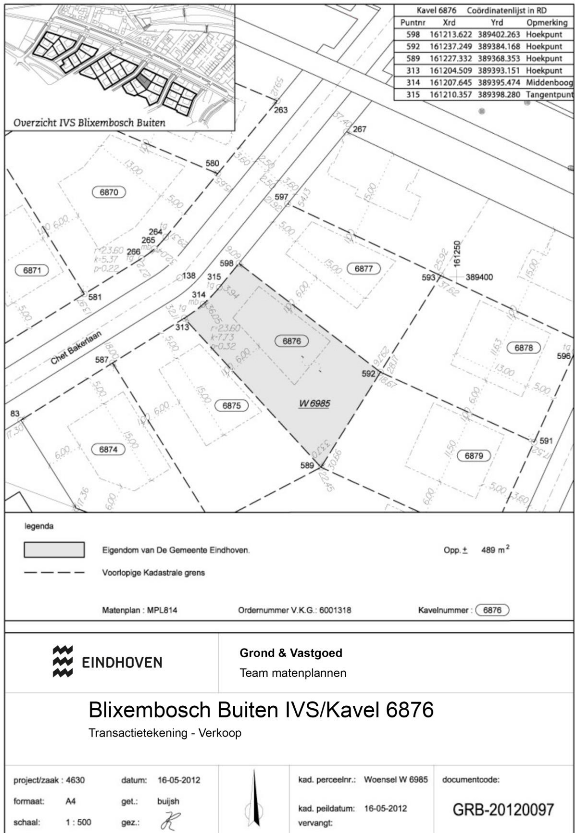
Afbeelding 3: Kadastrale verkooptekening van kavel 6876.
