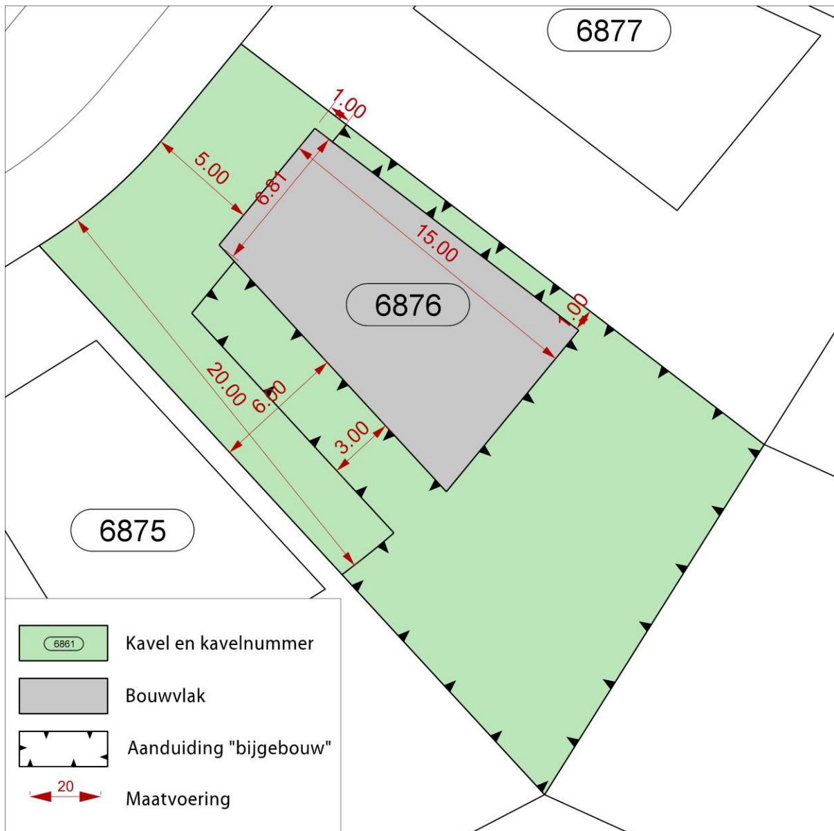
Afbeelding 4: bebouwinggrenzen geprojecteerd op kavel 6876.
