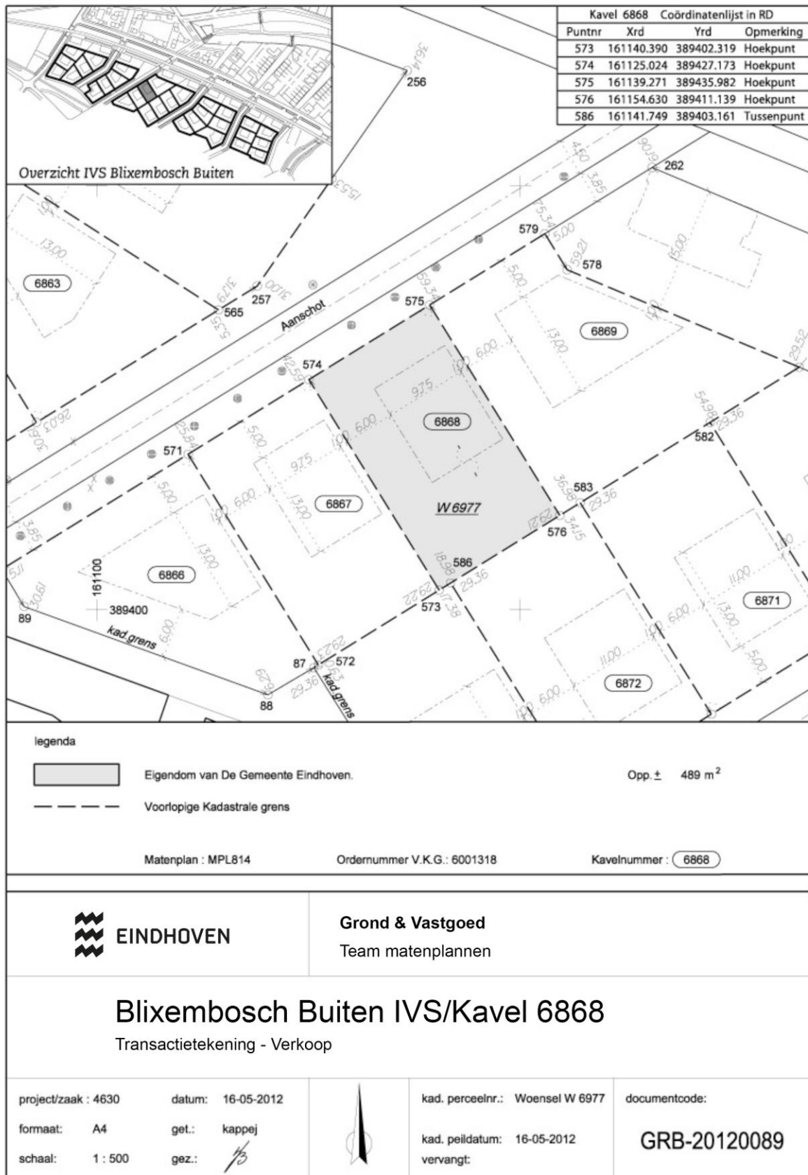
Afbeelding 3: Kadastrale verkooptekening van kavel 6868.
